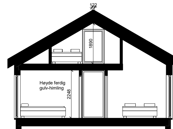
SNITT 1 1 : 100
