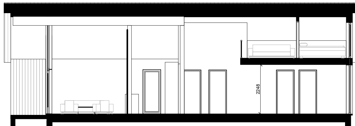
SNITT 3 1 : 100
