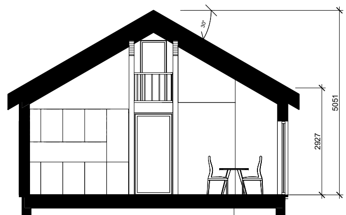
SNITT 2 1 : 100
