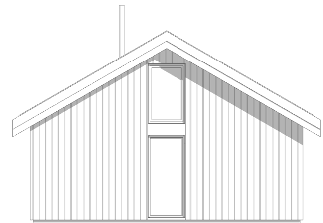
Fasade 4 1 : 100
