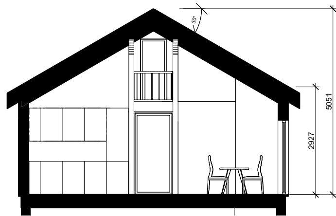
SNITT 1 1 : 100
